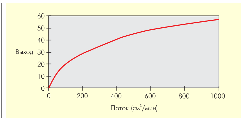
Рисунок 2 Типовая характеристика преобразования датчика с диапазоном 1 л/мин
