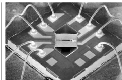
Рисунок 1 Структура чувствительного элемента датчиков расхода газа Honeywell
